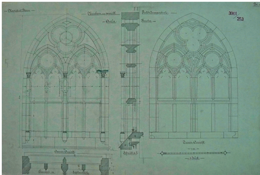
Il. 6. Projekt okien, APT, AmT, T 47, K. 58
